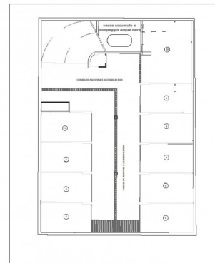
PIANTA PIANO AUTOCARROZZA
