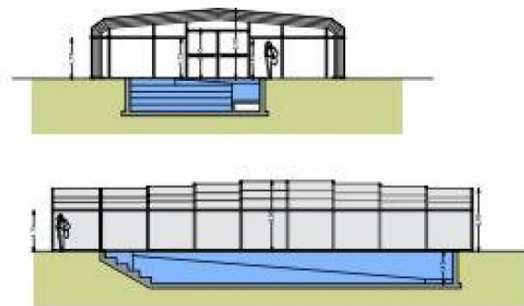
SEZ. LONGITUDINALE
